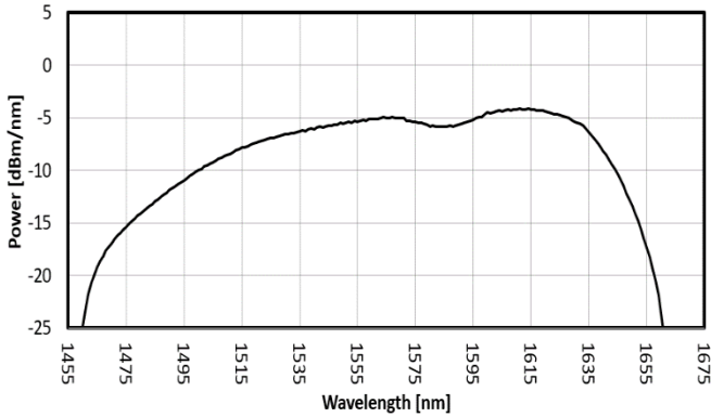
FIG. 1: ISB2 SPECTRUM
