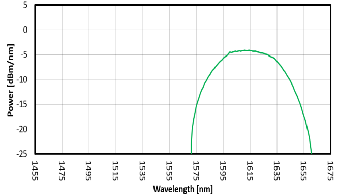
FIG. 2: SLED 1 SPECTRUM
