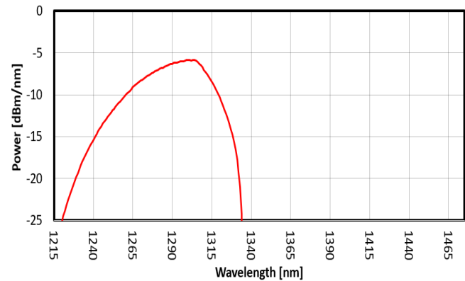
FIG. 4: SLED 3 SPECTRUM
