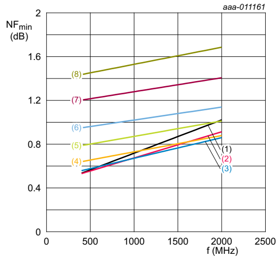
V CE = 8 V; T amb = 25 °C; Γ S = Γ opt . (1) I C = 1 mA (2) I C = 2 mA (3) I C = 3 mA (4) I C = 5 mA (5) I C = 10 mA (6) I C = 15 mA (7) I C = 25 mA (8) I C = 35 mA
