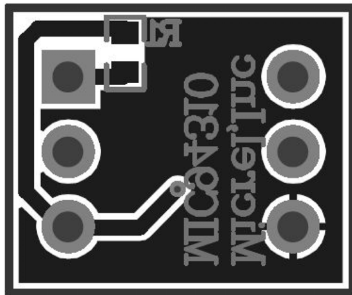
Bottom Layer
