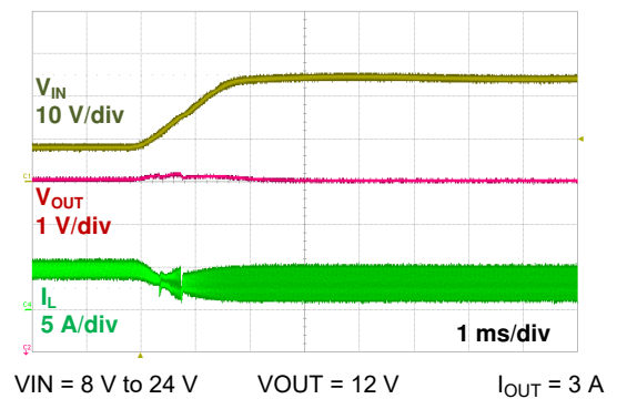
图 6-18. Line Transient
