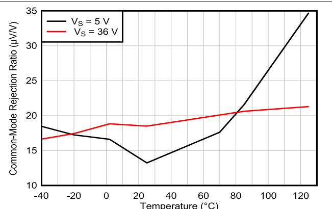
图 6-10. 共模抑制比与温度间的关系 (dB)
