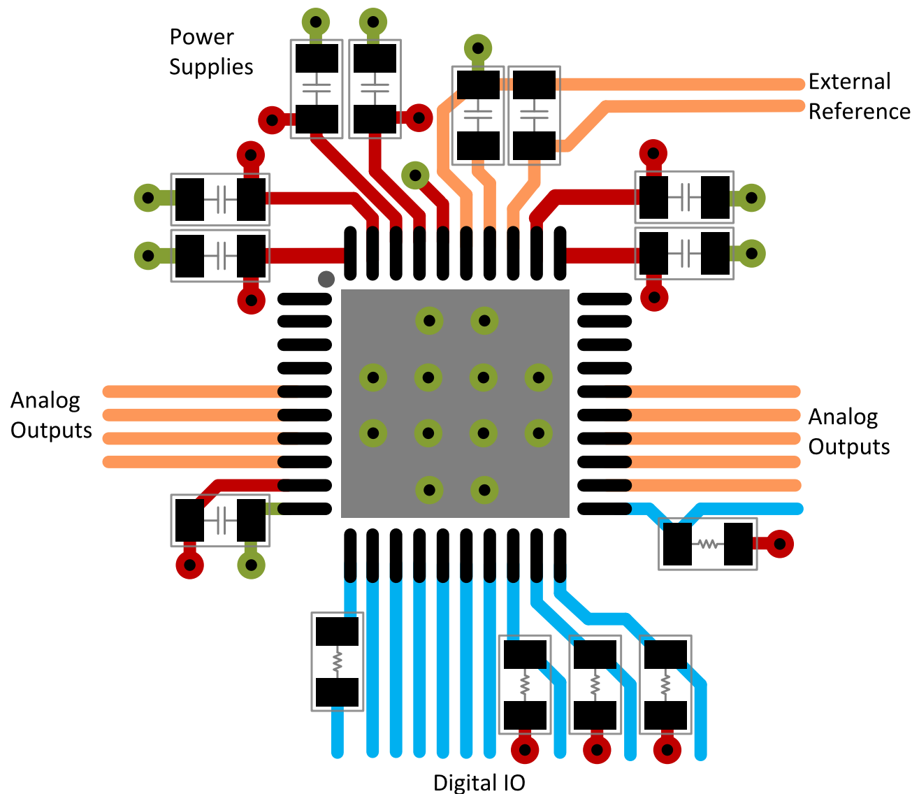
图 70. Example Layout
