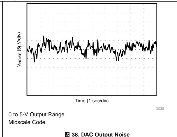
图 38. DAC Output Noise
