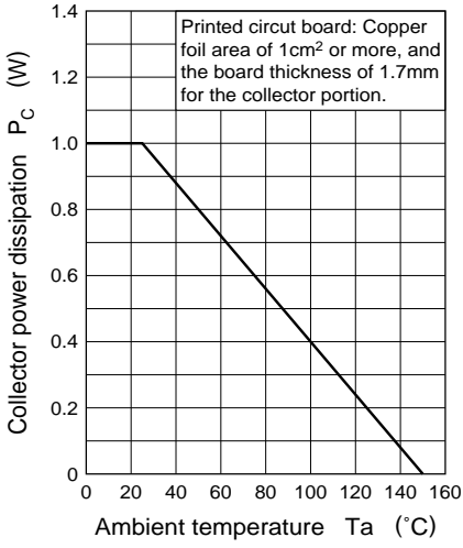
P_C - T_a
