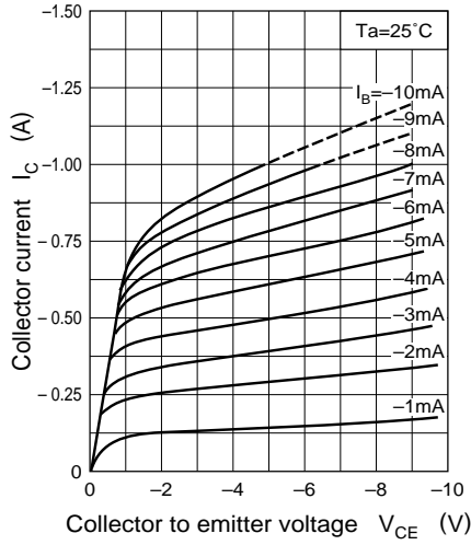
I_C - V_{CE}
