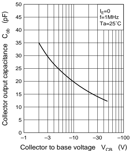
C_{ob} - V_{CB}
