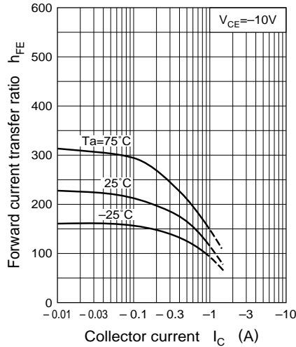
h_{FE} - I_C
