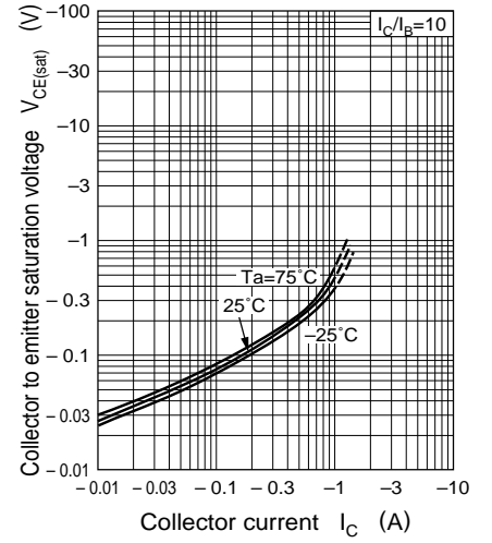
V_{CE(sat)} - I_C
