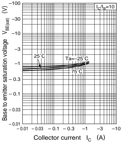
V_{BE(sat)} - I_C
