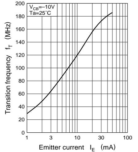
f_T - I_E
