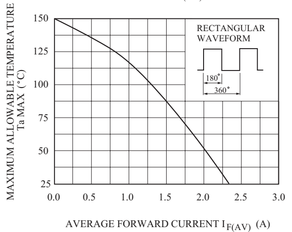
T_a - I_{F(AV)}
