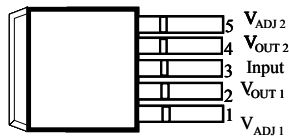
TO-263-5 Package
