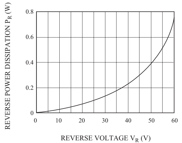
P_R - V_R
