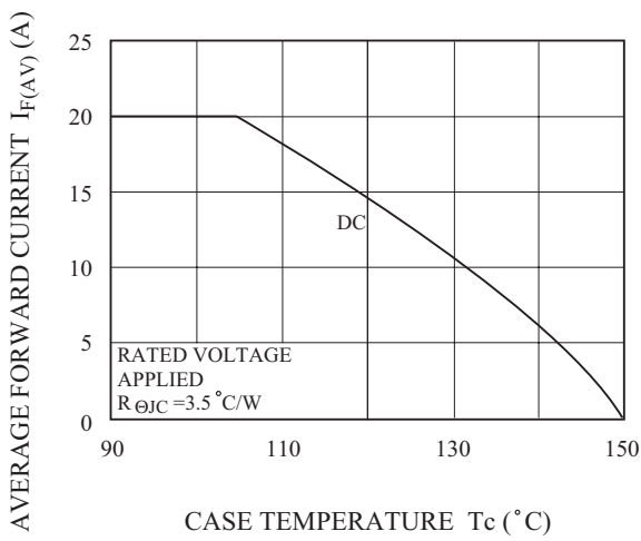
I_F - T_C
