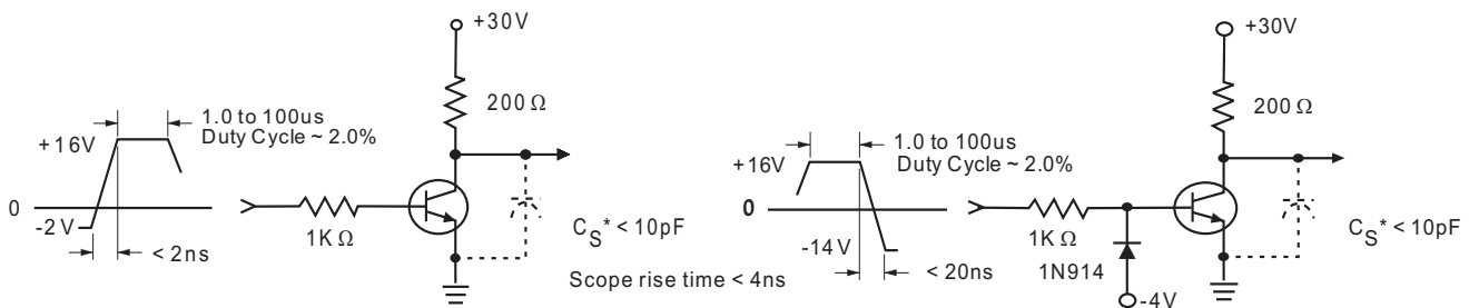
Fig. 1 Turn-On Time
