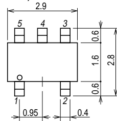
外形図 2171
