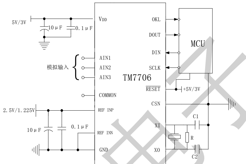
图 5 TM7706 的电路图
