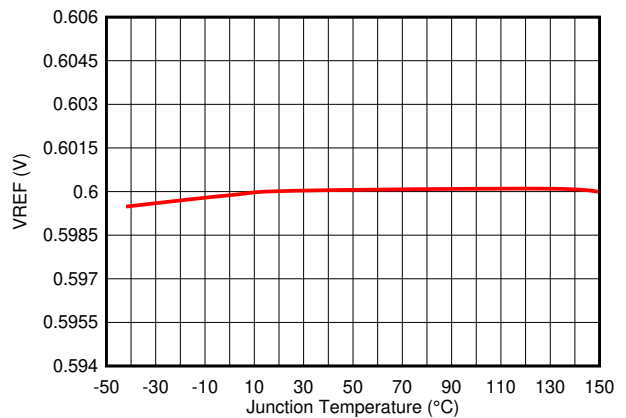
图 6-6. Vref
