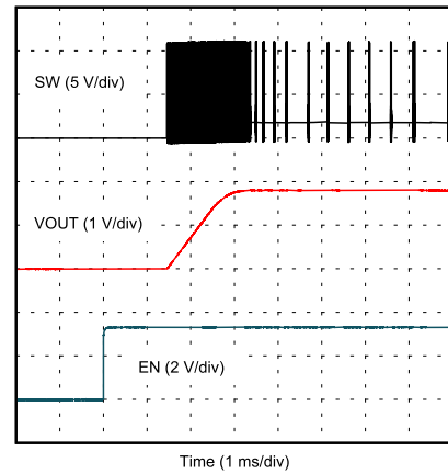
图 8-15. EN Start-Up
