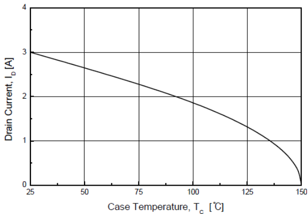
Fig. 9 I_D - T_C
