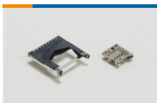
SD 卡连接器(1)
