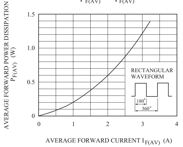
P_{F(AV)} - I_{F(AV)}
