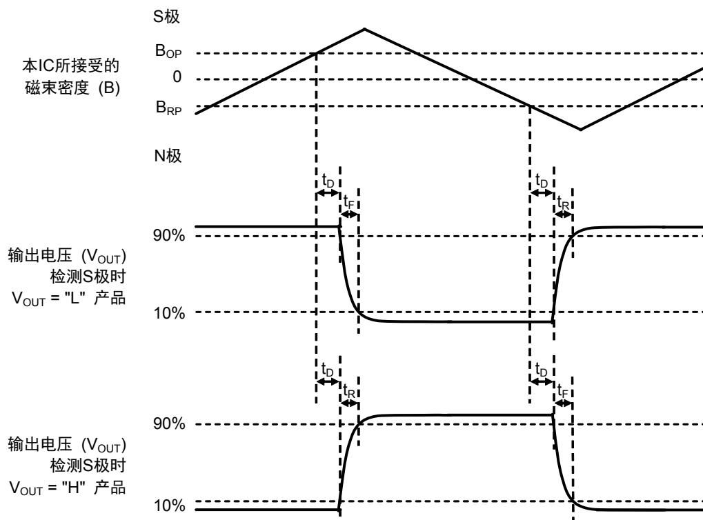
图3 工作时序
