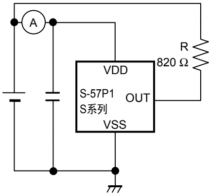
图4 测定电路1
