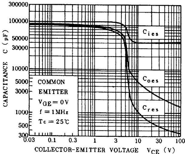
C - V_{CE}
