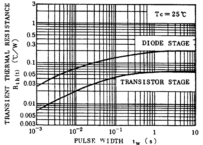
R_{th}(t) - t_w
