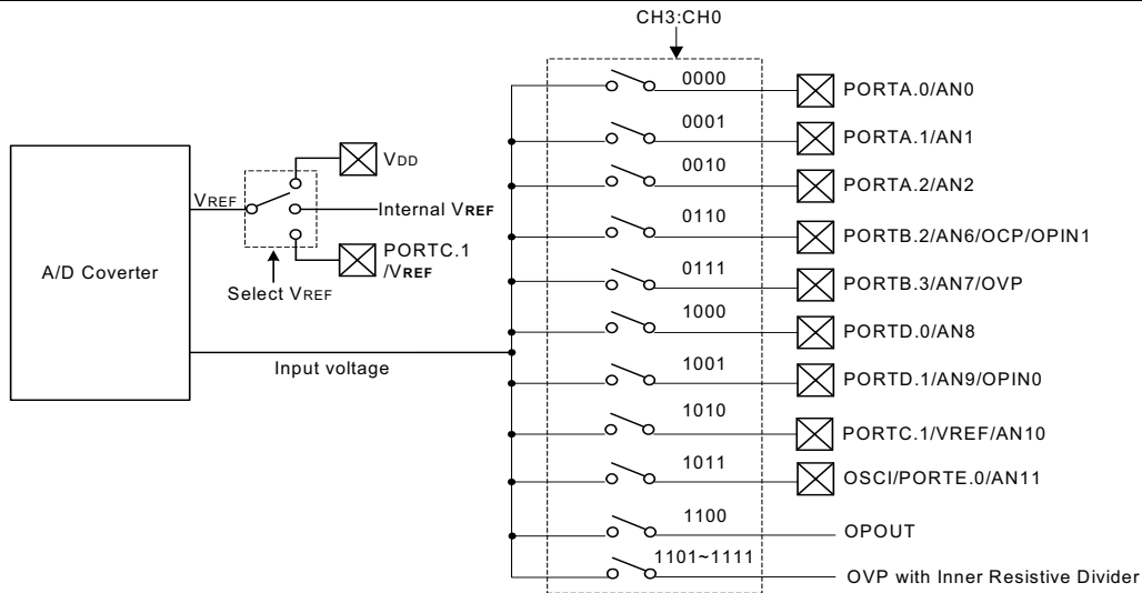
模/数转换器示意图
