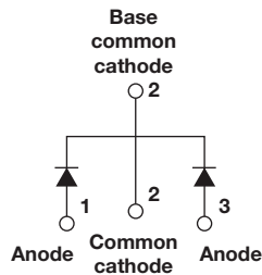
TO-263AB (D 2 PAK)
