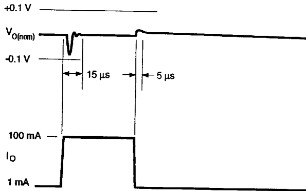
Dwg. WP-028-2
