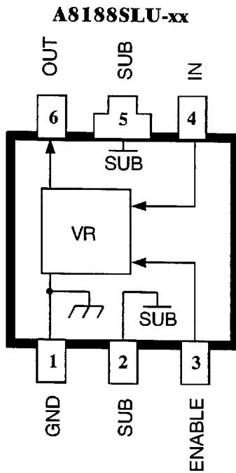
Dwg. PS-021-2
