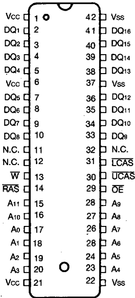
(SOJ)
