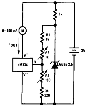
0°C–100°C Thermometer
