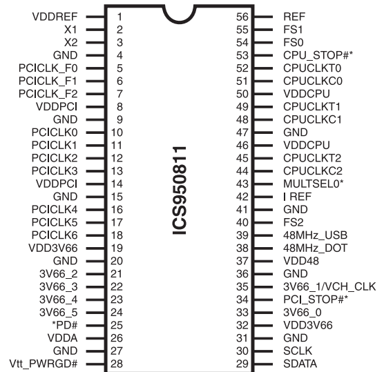
56 pin SSOP/TSSOP
