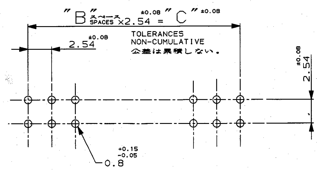
プリント基板推奨取付穴位置 RECOMMENDED HOLE LAYOUT
