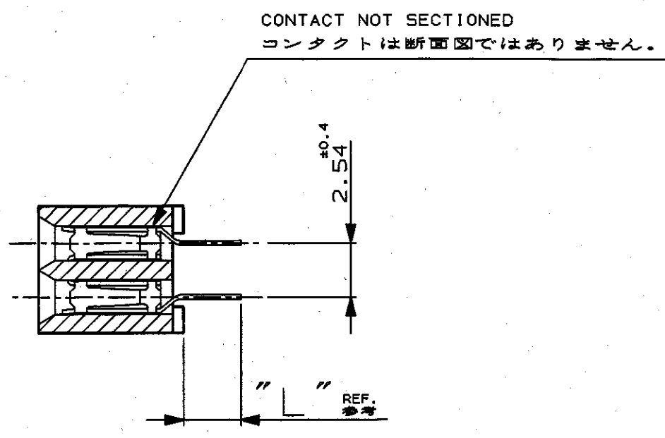
断面 "X-X" SECT "X-X"
