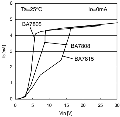
Fig.16 Vin - Ib
