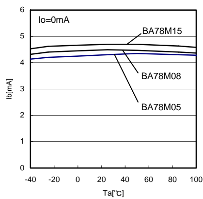
Fig.11 Ta - Ib
