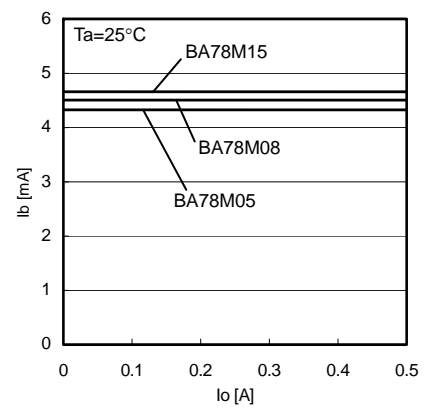
Fig.12 Io - Ib
