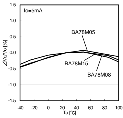
Fig.10 Ta - Vo
