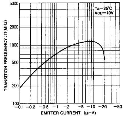
Fig.8 利得帯域幅 —エミッタ電流特性
