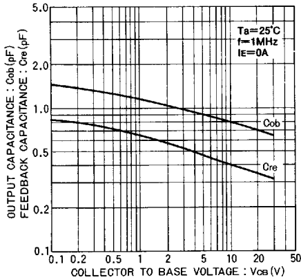
Fig.7 出力容量・帰還容量—電圧特性
