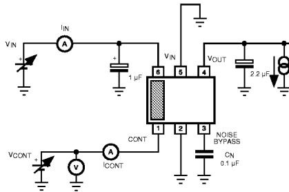
SOT-23L
