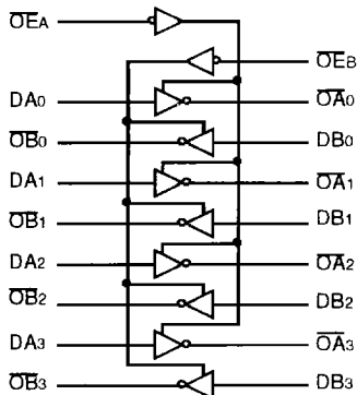
IDT54/74FCT240
