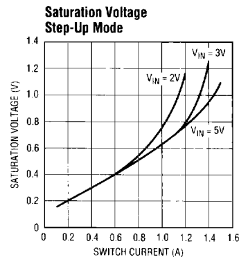
LT1111 • TPC06
