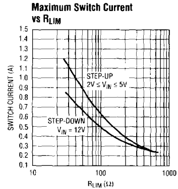
LT1111 • TPC 12
