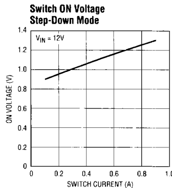
LT1111 • TPC08
