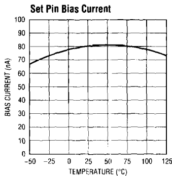
LT1111 • TPC 13
