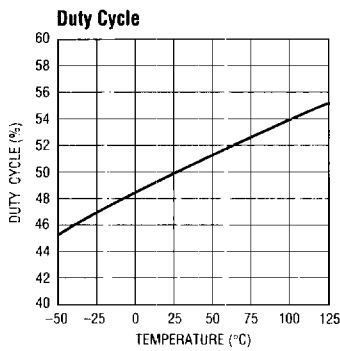
LT1111 • TPC04
