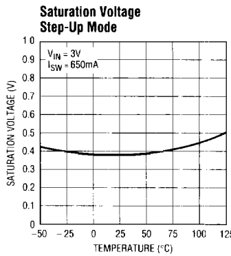
LT1111 • TPC05
