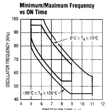
LT1111 • TPC09
