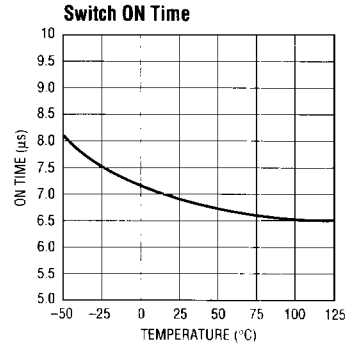
LT1111 • TPC03
