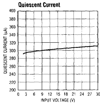
LT1111 • TPC 9
