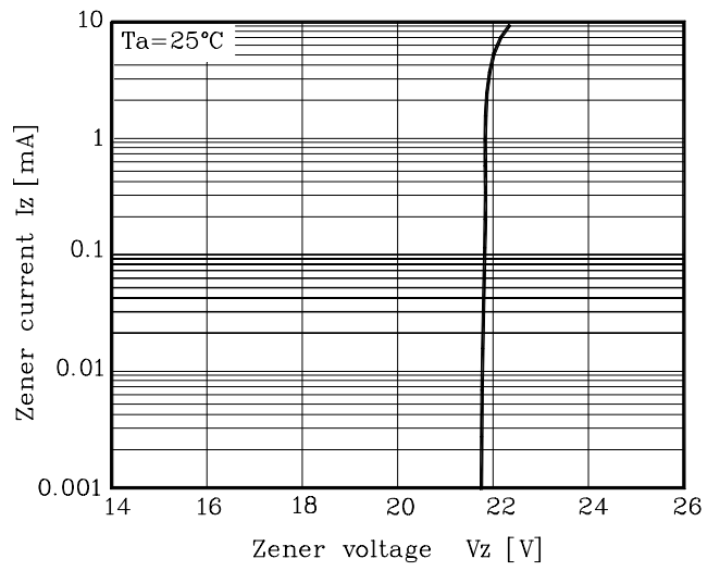
Fig. 2 I_Z - V_Z
