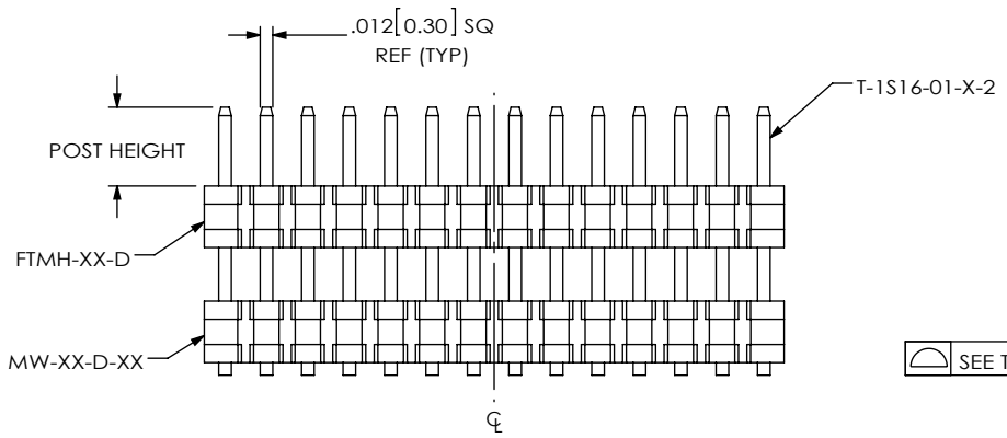
FIG 1 MW-14-03-X-D-180-075 SHOWN
