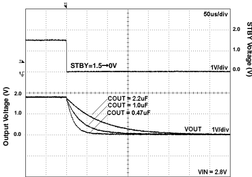
Fig 26. Discharge Time
