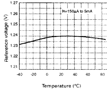
Temperature (°C) Temperature Drift
