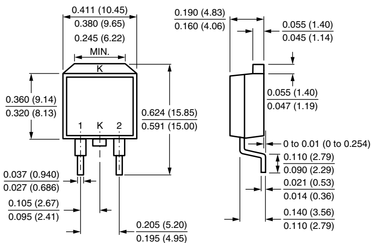
TO-263AB
