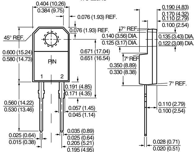
ITO-220AC
