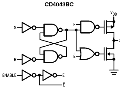
CD4043BC
