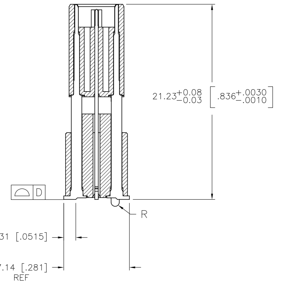
SECTION A-A
