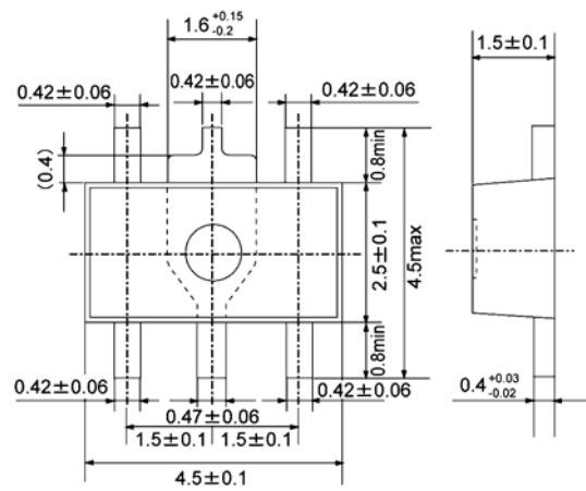
SOT-89-5
