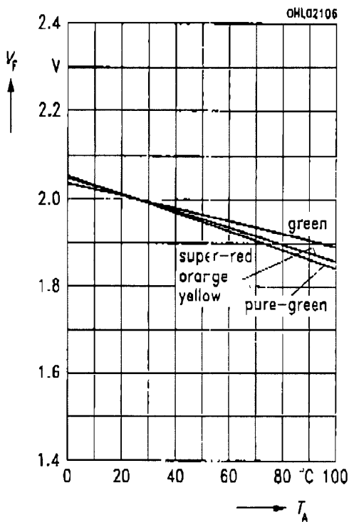
Durchlaßspannung V_F = f(T_A) Forward voltage I_F = 10 \text{ mA}
