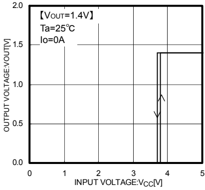
Fig.46 Vcc-Vout
