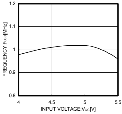
Fig.10 V CC -F osc
