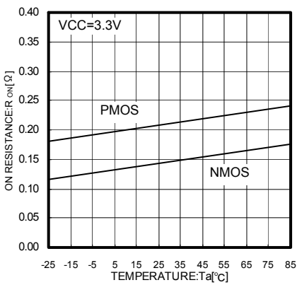
Fig.67 Ta-Ronp, Ronp
