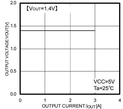
Fig.48 Iout-Vout
