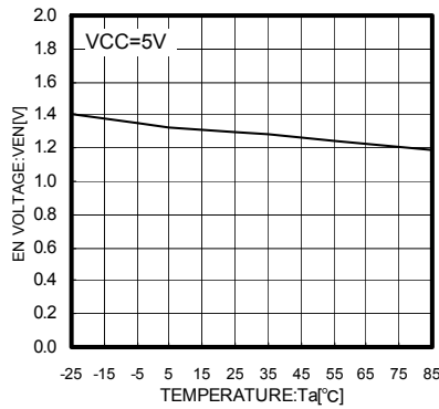
Fig.8 Ta-Ven
