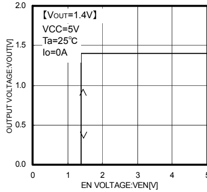
Fig.47 Ven-Vout
