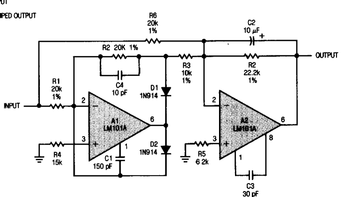
Precision Rectifier
