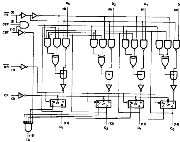
'LS161A
