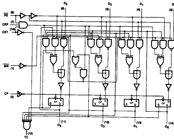
'LS162A
