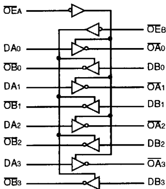
IDT54/74FCT240
