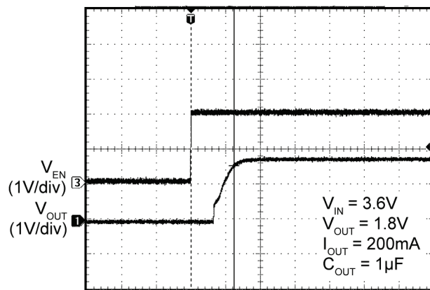
Enable Turn-On
