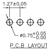
P.C.B. LAYOUT
