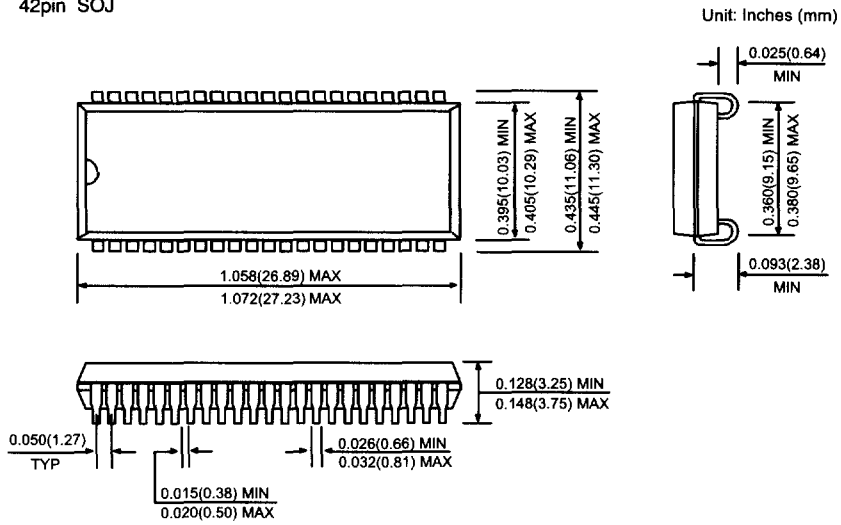
42pin SOJ
