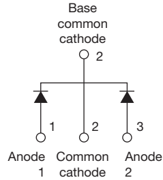
VS-MURB1620CTPbF
