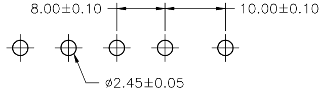
P.C.B LAYOUT
